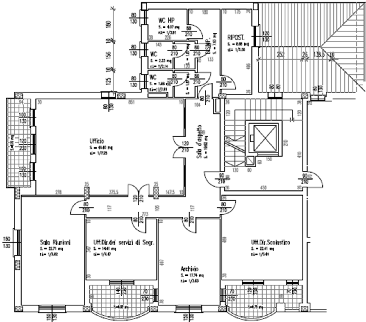
PLANIMETRIA PIANO PRIMO
